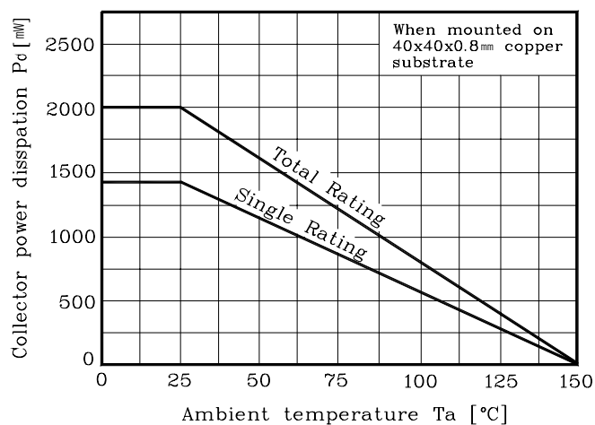
Fig. 1 P_C - T_a
