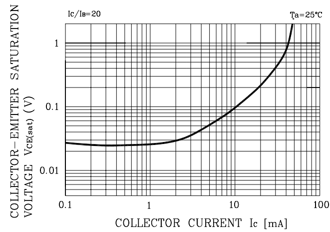
Fig. 2 V_{CE(sat)} - I_C
