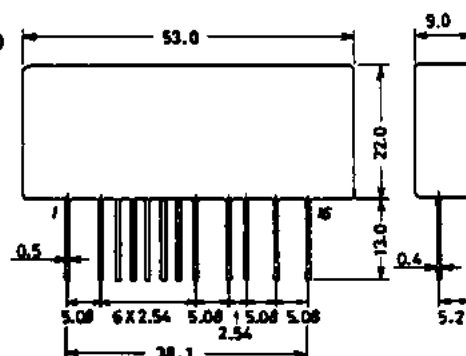
外形図 4056 (unit: mm)
