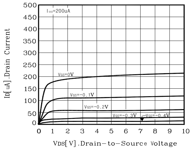
Fig. 2 I_D - V_{DS}
