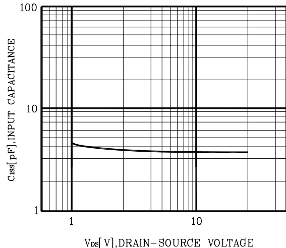
Fig. 6 C_{iss} - V_{DS}
