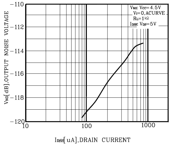
Fig. 9 V_{NO} - I_{DSS}
