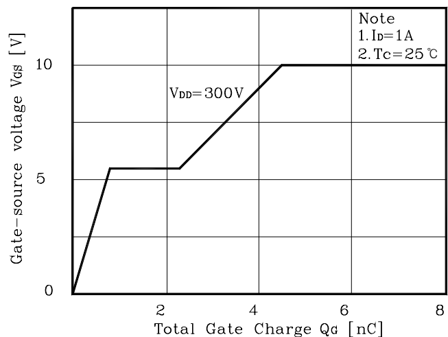
Fig. 6 V_{GS} - Q_g
