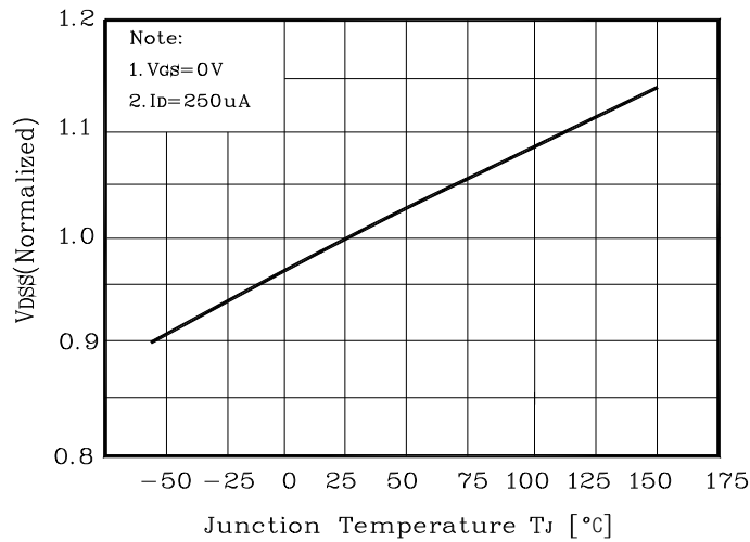
Fig. 7 V_{DSS} - T_J
