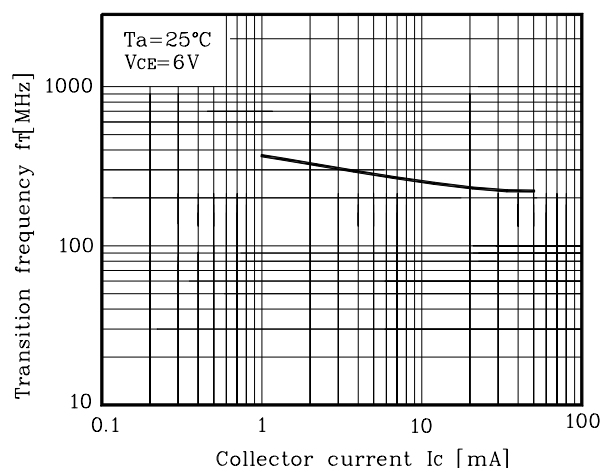
Fig. 4 f_T - I_C
