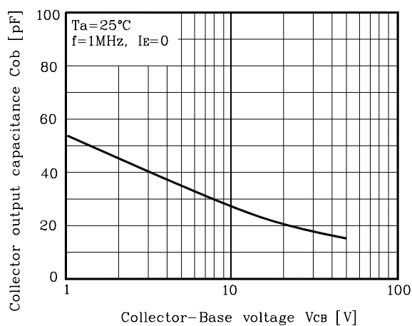
Fig. 5 C_{ob} - V_{CB}
