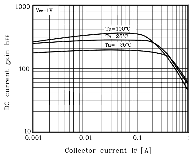
Fig. 6 h_{FE} - I_C
