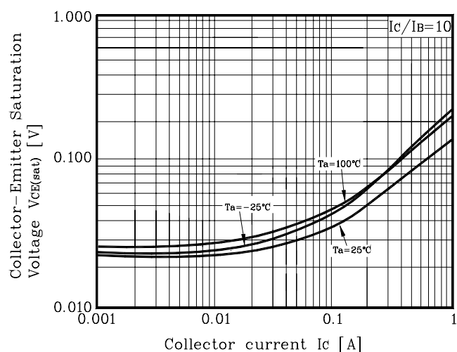
Fig. 5 I_C - V_{CE}
