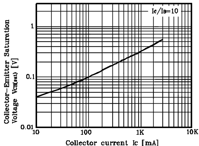
Fig. 2 V_{CE(sat)} - I_C
