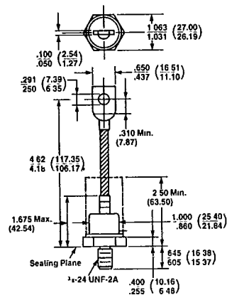
JEDEC DO-8
