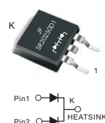
TO-263
