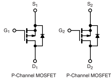
P-Channel MOSFET
