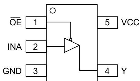
SOT23-5/SC70-5
