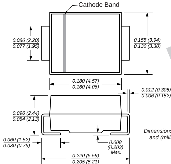
DO-214AA (SMBJ-Bend)
