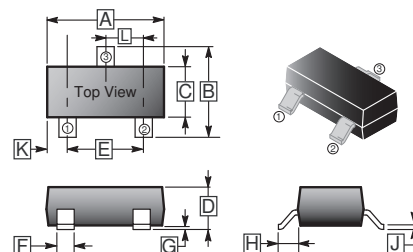
SC-59
