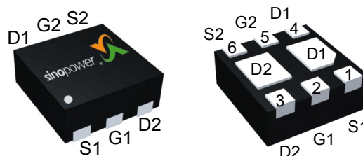
DFN2x2C-6_EP2
