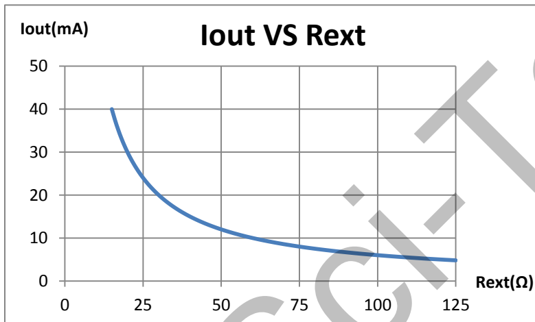
图 1. SM2082EAS 输出电流与 R_{EXT} 电阻关系曲线
