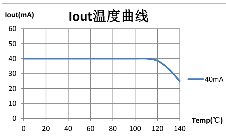
图 3. SM2082EAS 输出电流温度特性（注 8）
