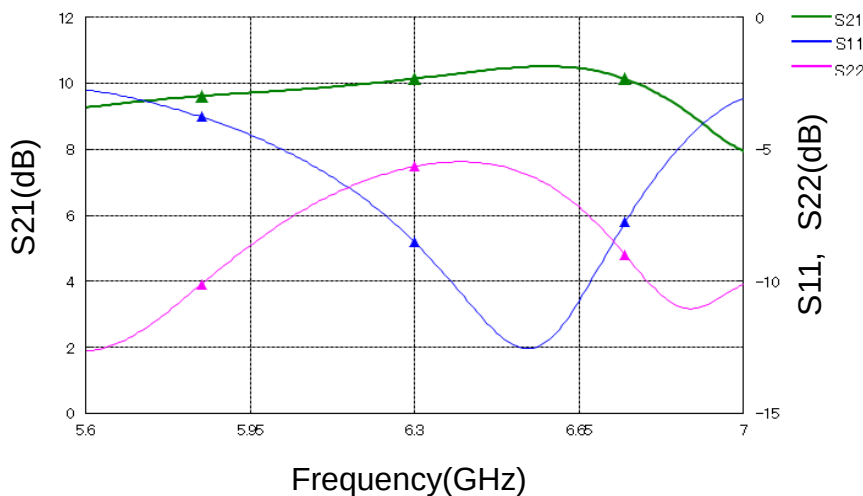
Log Mag
