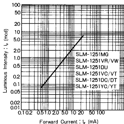
Fig.2 光度—順方向電流特性
