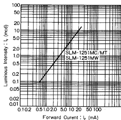
Fig.3 光度—順方向電流特性
