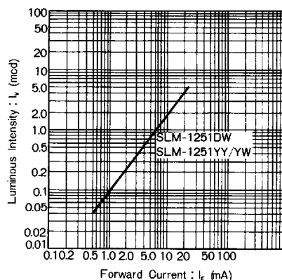
Fig.1 光度—順方向電流特性
