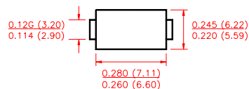
DO-214AB(SMC)
