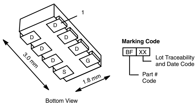
1206-8 ChipFET®
