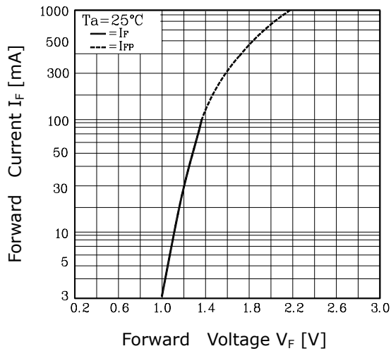
Fig. 1 I_F - V_F
