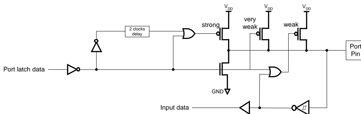
Quasi-bi Mode
