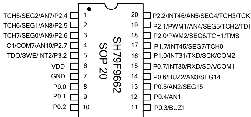
引脚配置图
