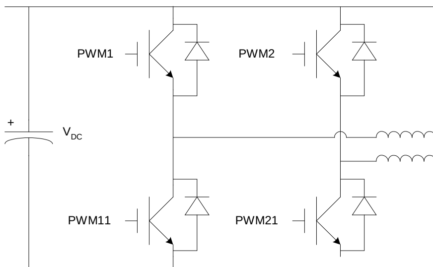
图8-1-15 PWM控制逆变桥示例图
