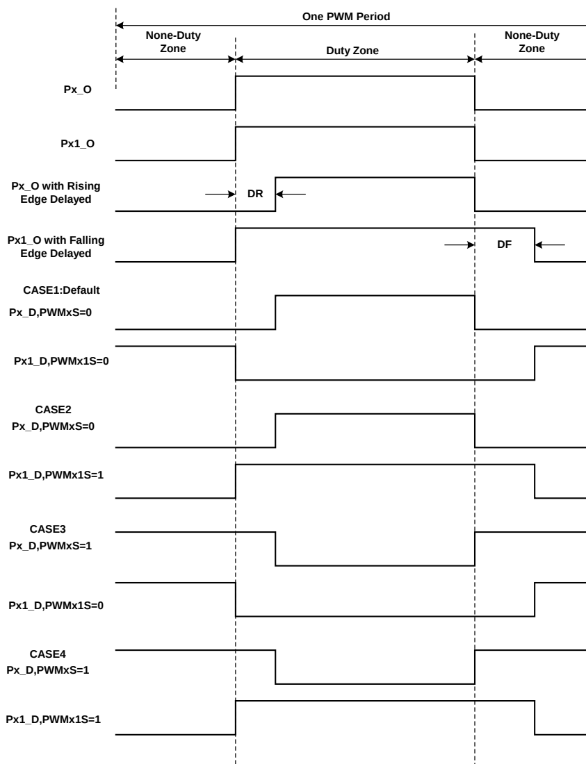
图8-1-13 不同极性设置下的死区波形
