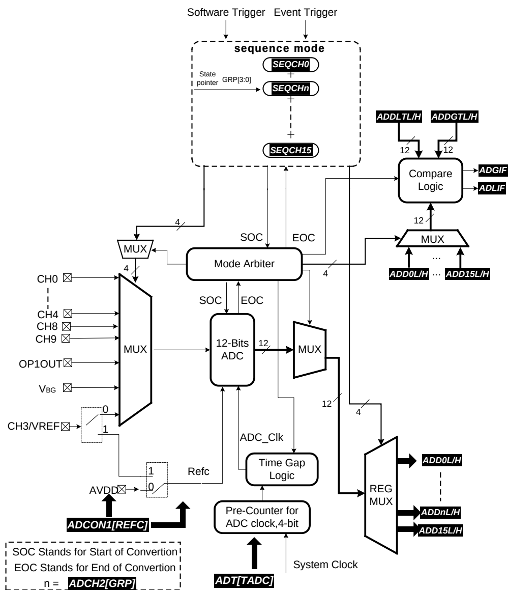
图8-4-1 ADC模块图
