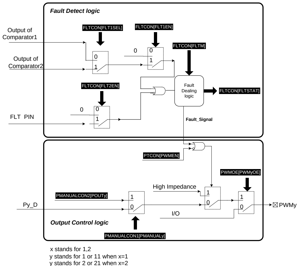
图8-1-14 输出控制与故障检测逻辑简图
