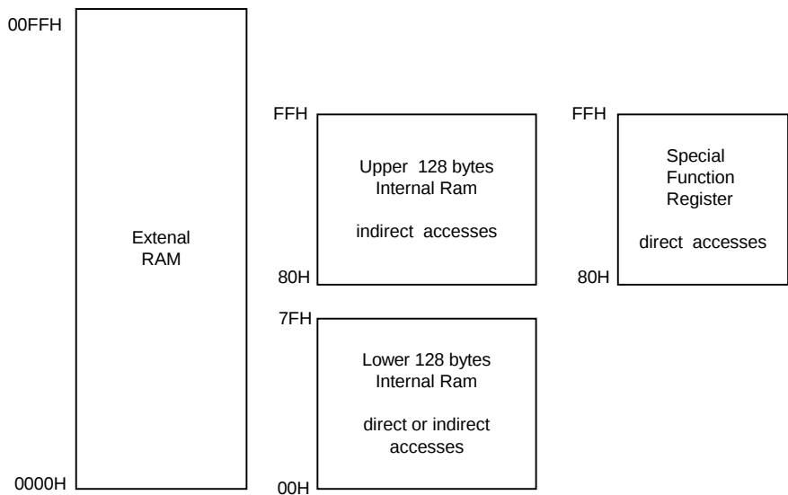
内部和外部RAM配置
