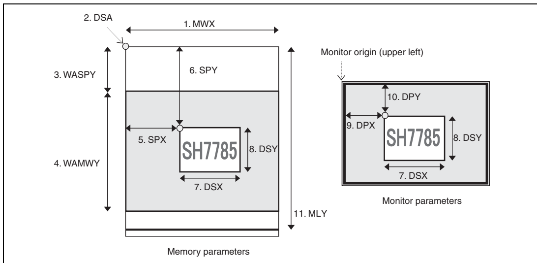
Figure 19.3 Parameters
