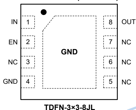
SGM2239-FIXQ (TOP VIEW)
