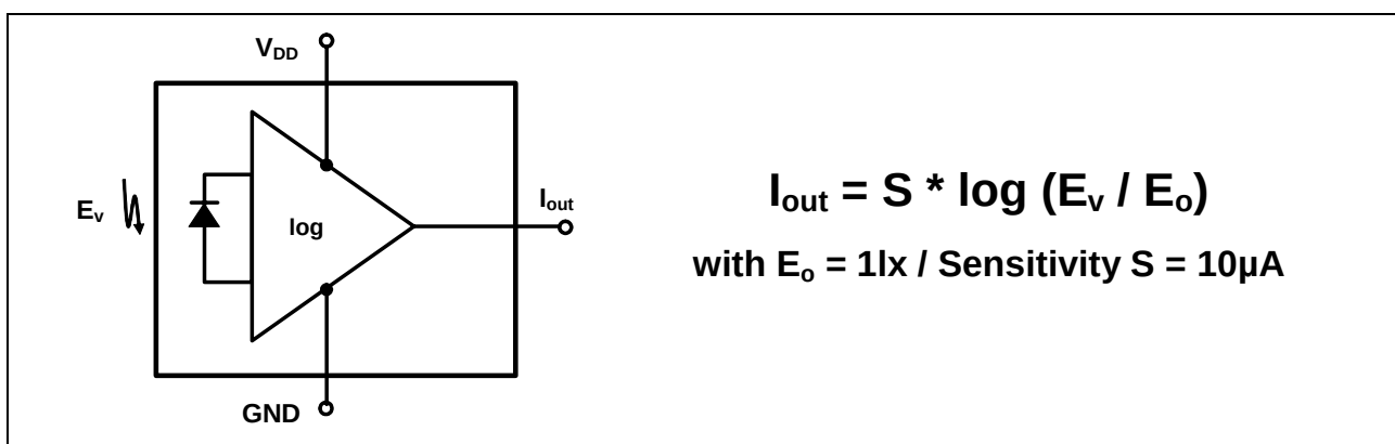
Figure 1 Ersatzschaltbild Circuitry
