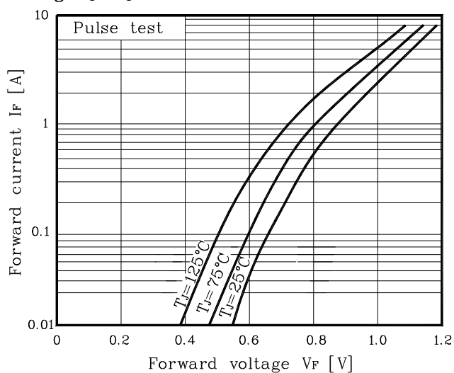
Fig.1 I_F - V_F
