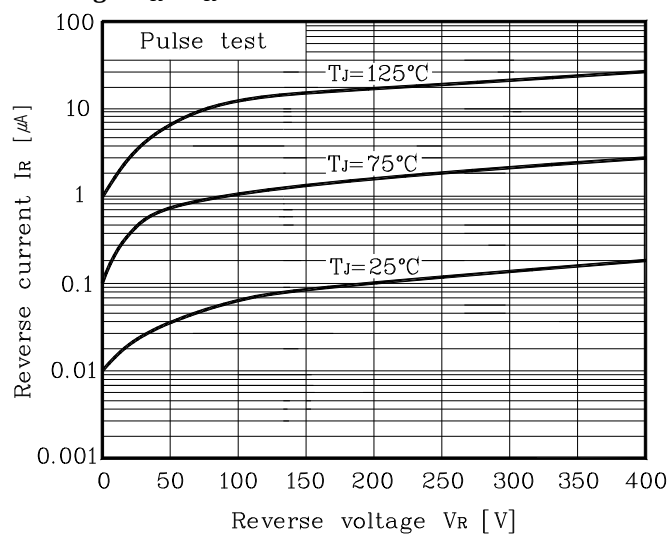
Fig. 2 I_R - V_R
