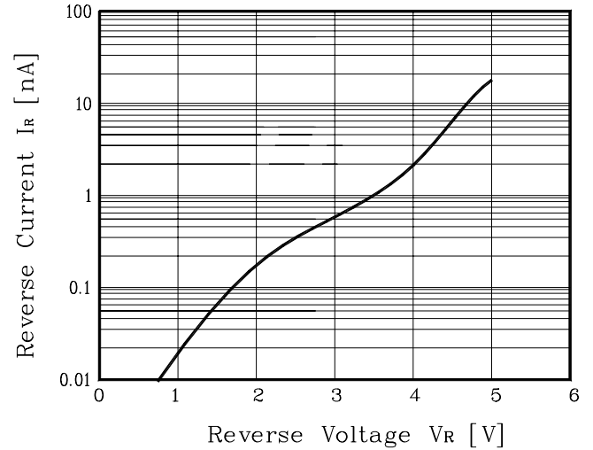
Fig. 2 I_R-V_R
