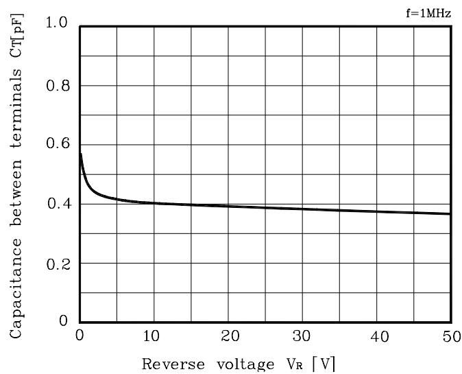
Fig. 3 C_T-V_R
