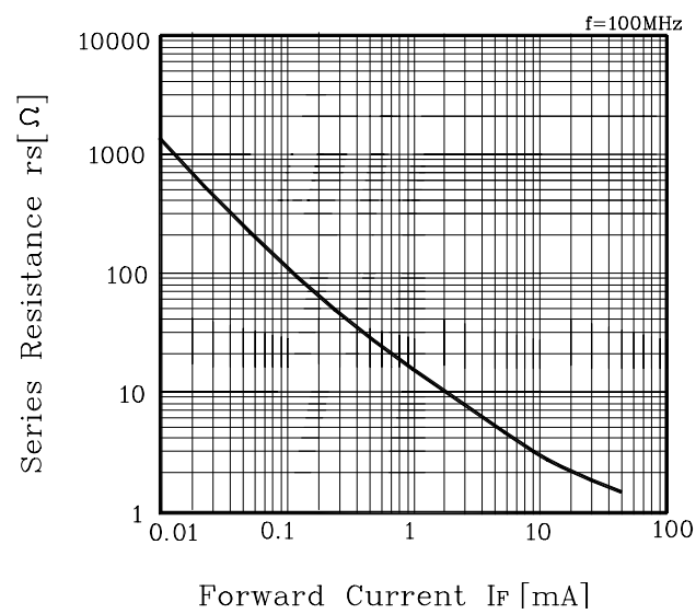
Fig. 4 r_s-I_F
