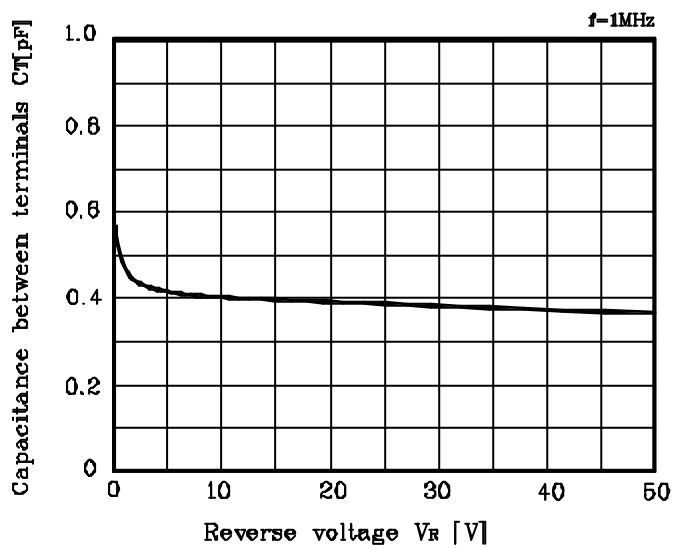
Fig. 3 C_T - V_R
