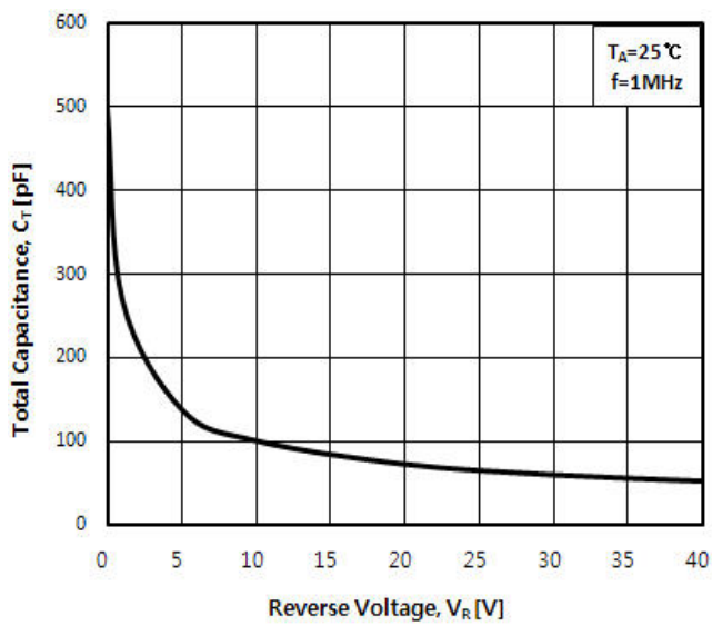
Fig. 3 C_T - V_R
