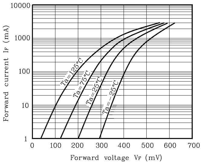
Fig. 1 I_F - V_F
