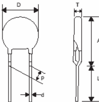
F type (Y kink lead)
