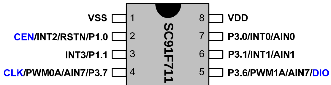
SC91F711管脚配置图
