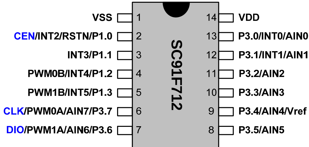
SC91F712管脚配置图
