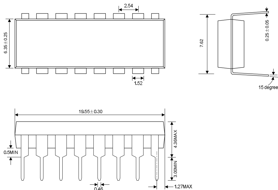
DIP-18-300-2.54
