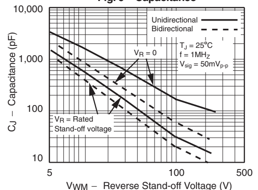
Fig. 6 - Capacitance
