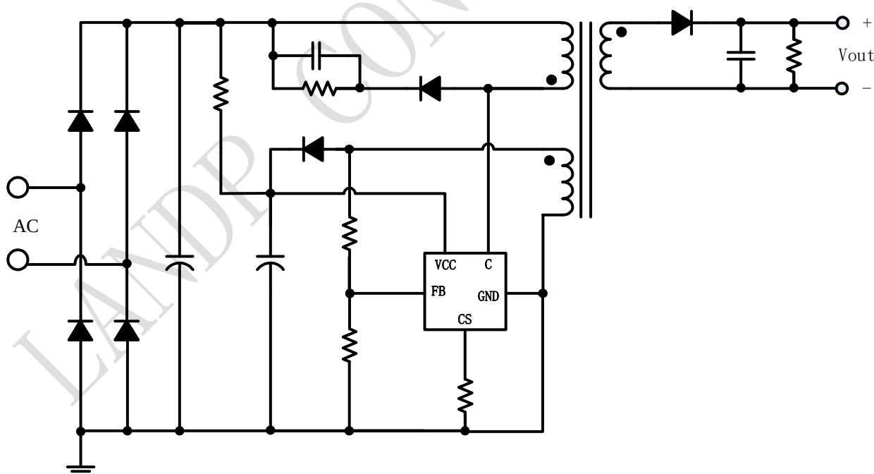
图 1 S9111A 典型应用图
