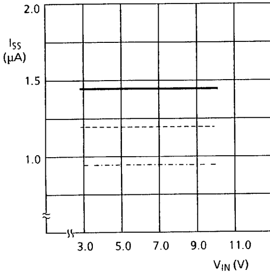
5.3 S-81225AG-RH-X
