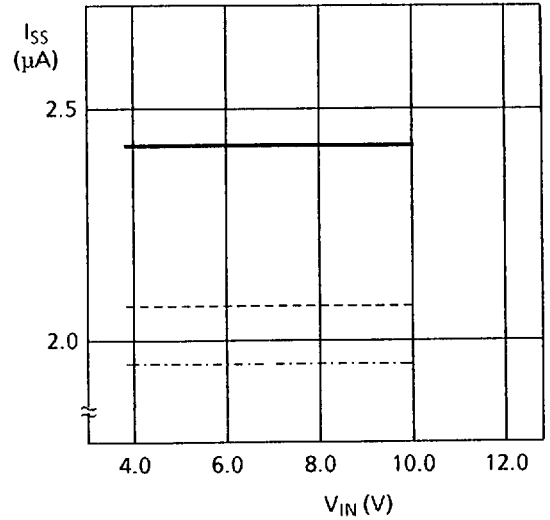
5.4 S-81230AG, S-81230AG-RB-X
