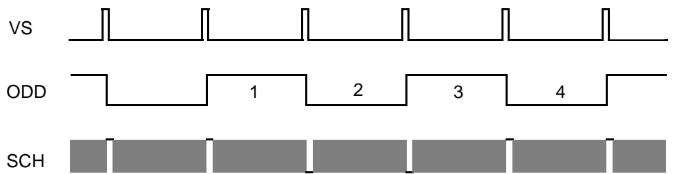
Truth Table
