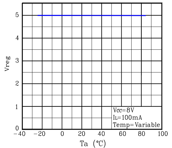
Fig. 16. T_a vs V_{reg}
