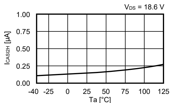
4. 14 I CAS2H vs. Ta
