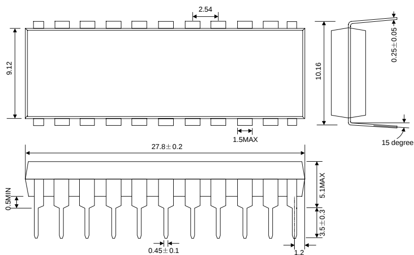
DIP-22-400-2.54
