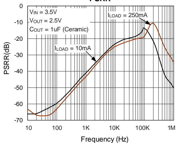
PSRR
