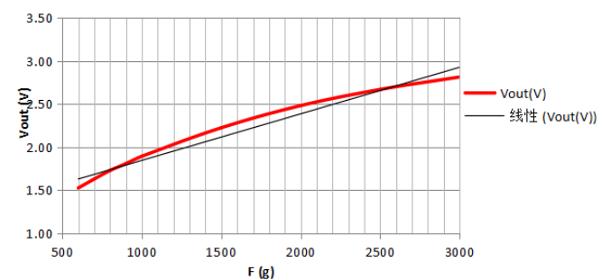
Vout(V)
