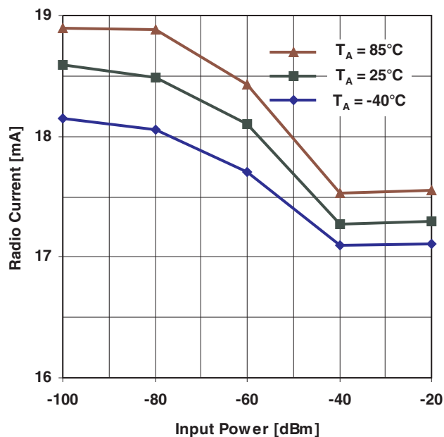
500 kBaud MSK
